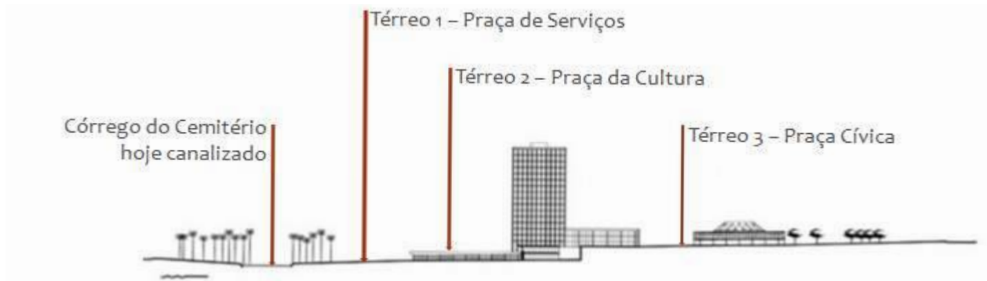
Corte geral do Centro Cívico de Santo André. Fonte: ANELLI, R.; GUERRA, A.; KON, N., Rino Levi: arquitetura e cidade. 2001, p.255.
