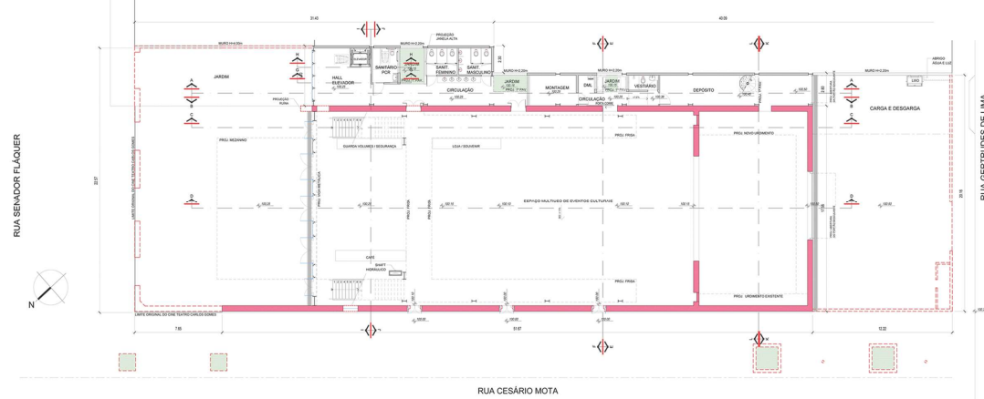
PLANTA BAIXA - Pavimento Térreo
