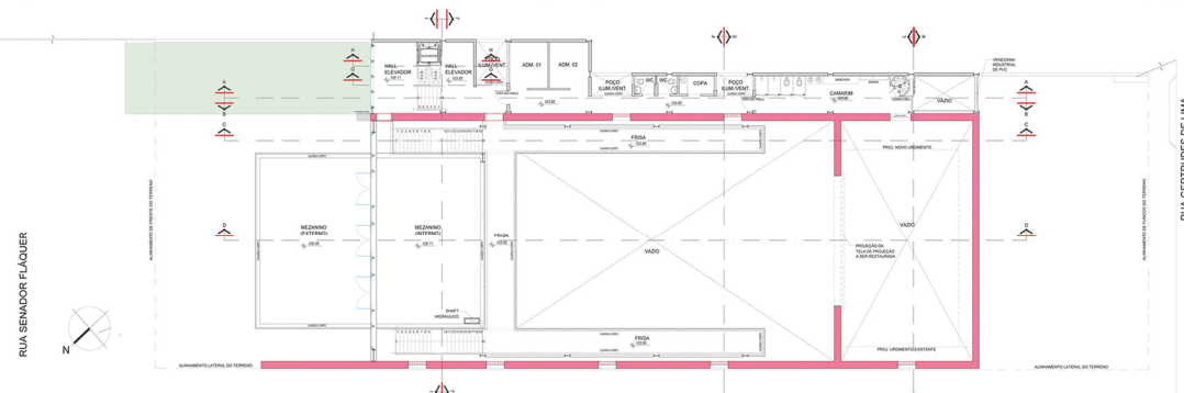
PLANTA BAIXA - 1o. Pavimento
