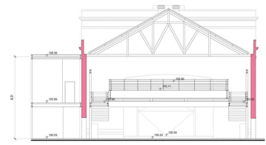
CORTE J-J
