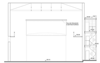
CORTE L-L
