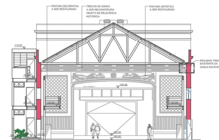
CORTE - BOCA DE CENA
