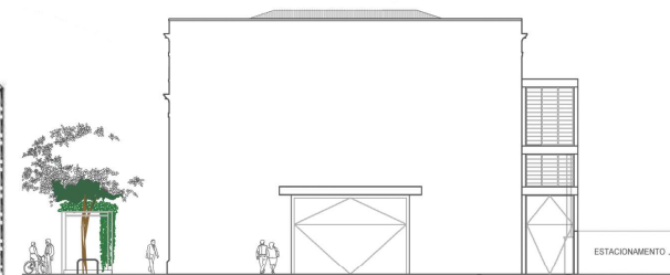
ELEVAÇÃO POSTERIOR - Rua Gertrudes de Lima
