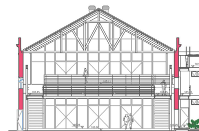
CORTE - FRISAS
