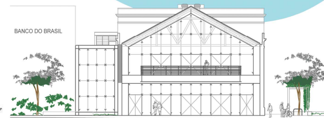
ELEVAÇÃO FRONTAL - Rua Senador Fláquer
