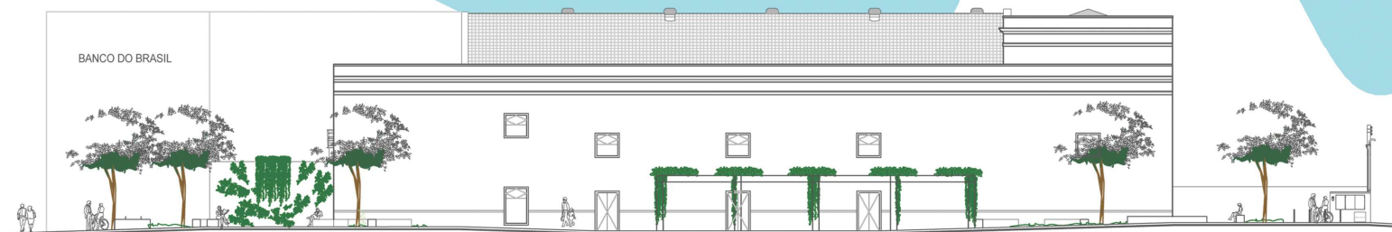
ELEVAÇÃO LATERAL - Rua Cesário Mota
